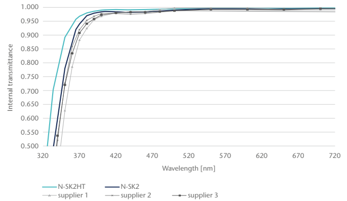
N-SK2HT, n_d = 1.60738 , v_d = 56.65
